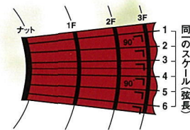
どの弦でもスペック上のスケール値と一致する
